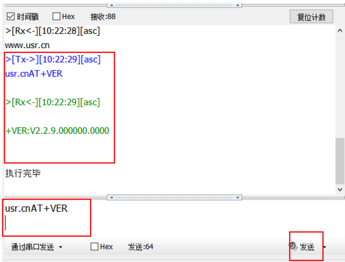
图 22 设置软件示意图
