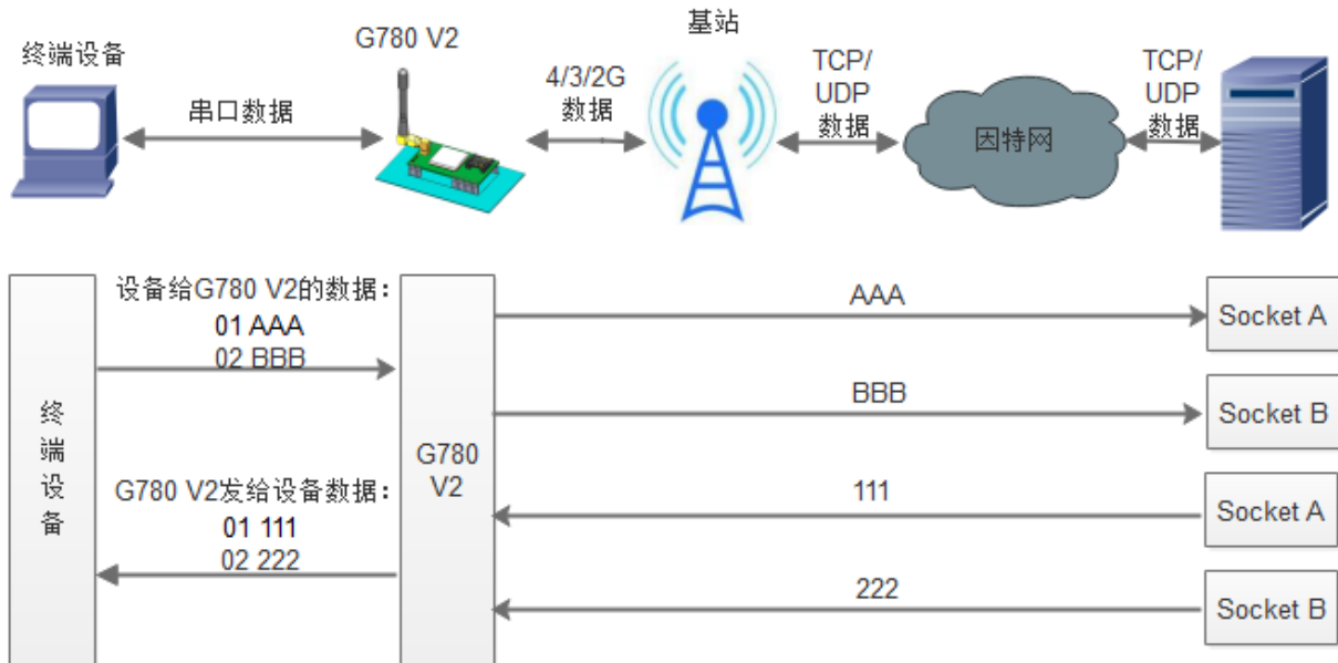
图 16 套接字分发协议示意图
