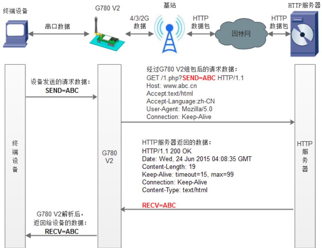
图6 HTTPD Client 模式示意图
