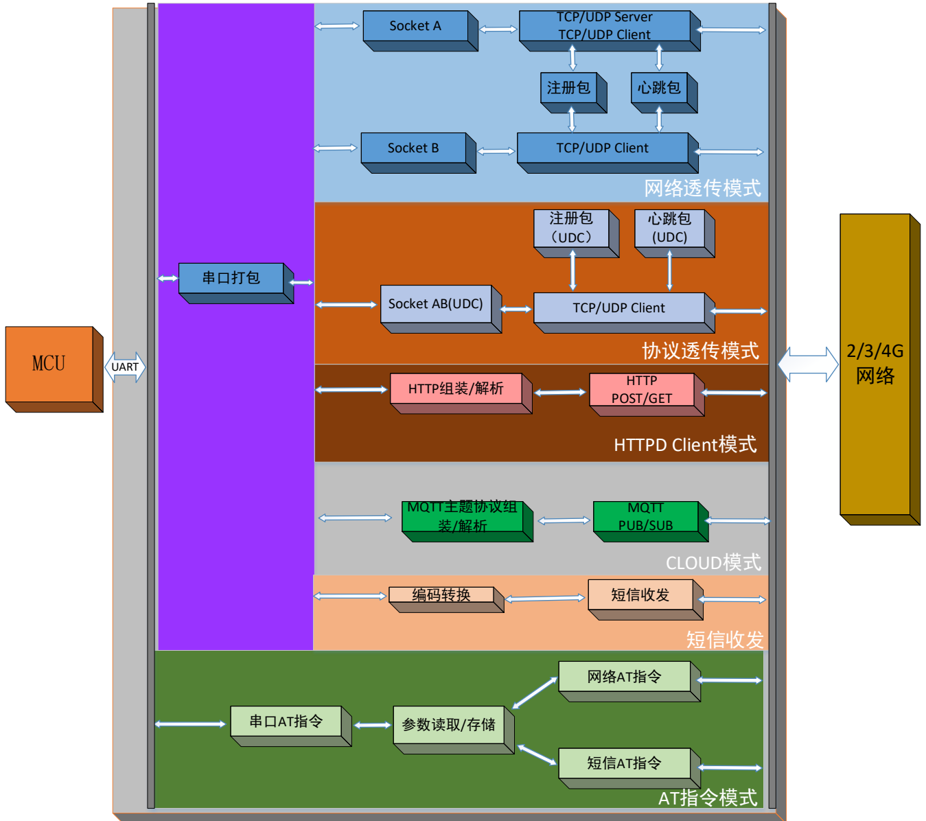
图 1 功能框图
