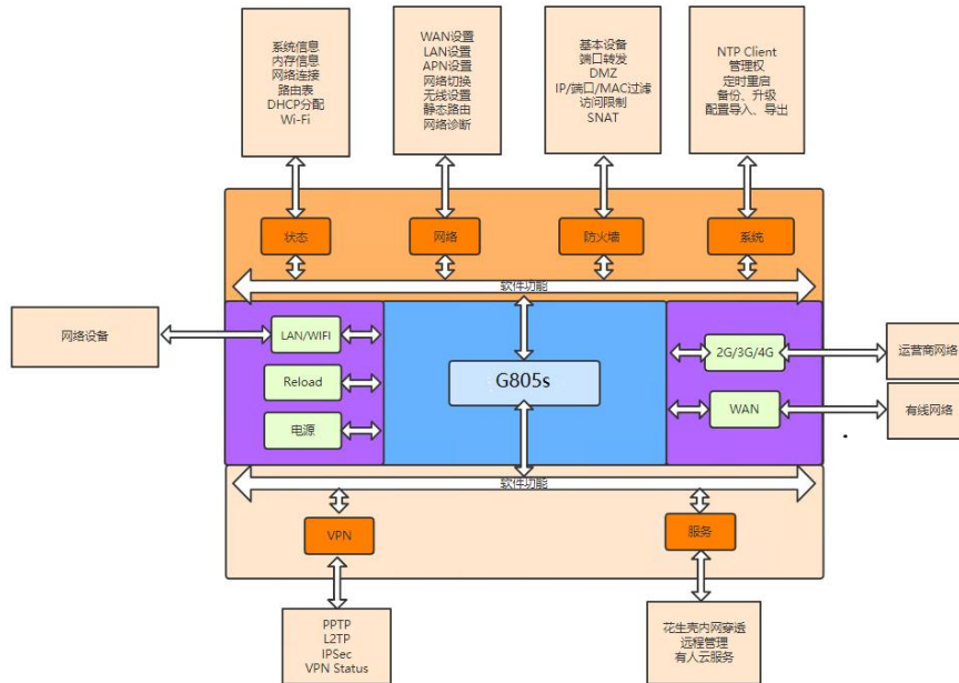
图 3 功能框图
