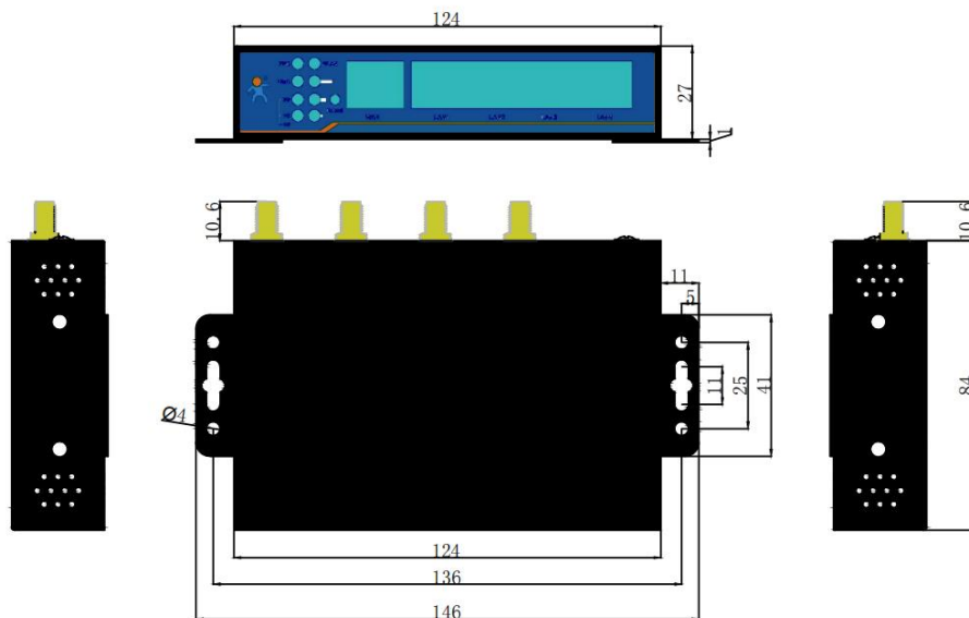
图 2 USR-G805s 外观尺寸图
