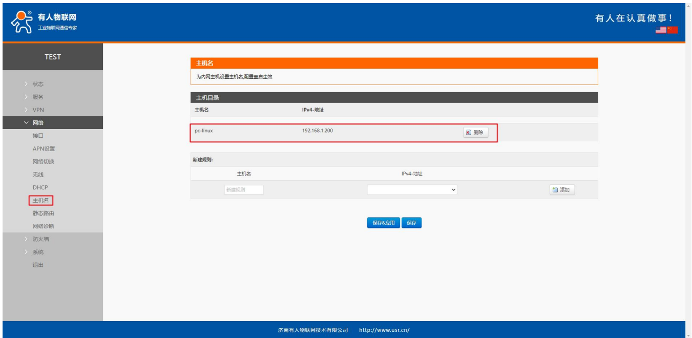
图 33 主机名页面
