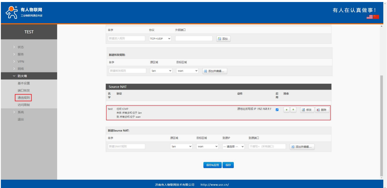
图 55 NAT 设置三
