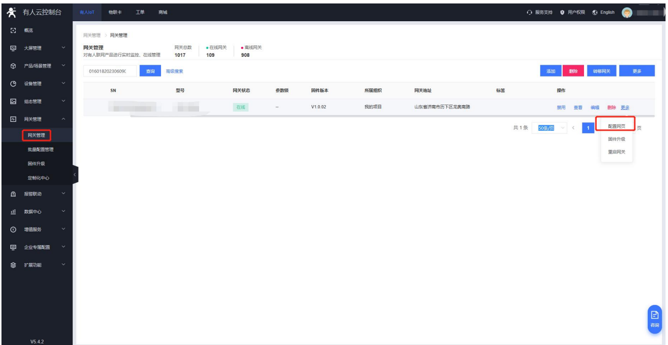
图 69 配置网页（一）
