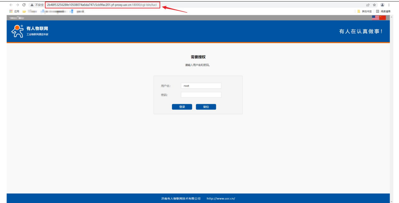
图 70 配置网页（二）
