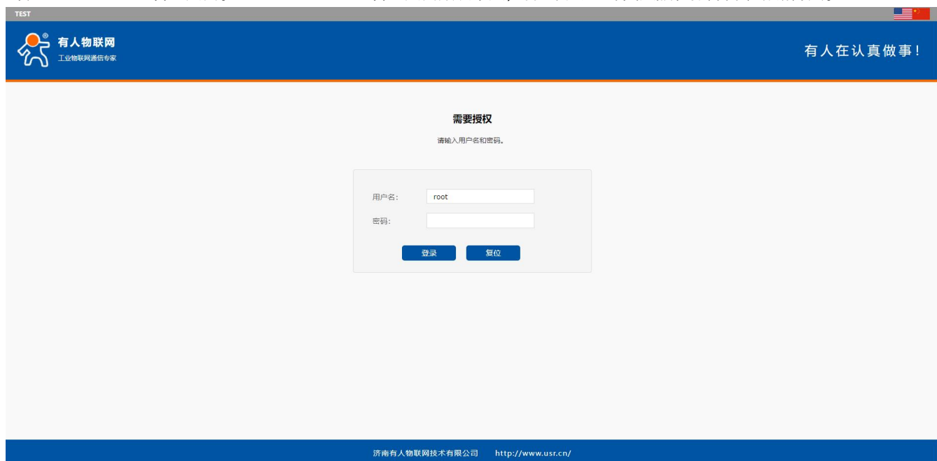
图 4 登录首页
