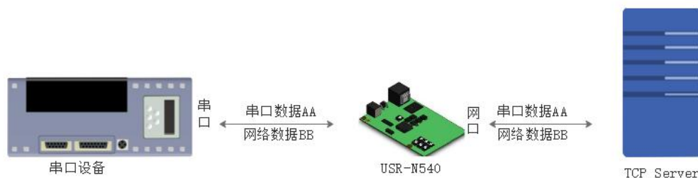
图 14 TCP Client 模式说明
