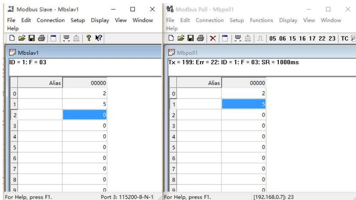
图 59 Modbus RTU 转 Modbus TCP 转换结果
