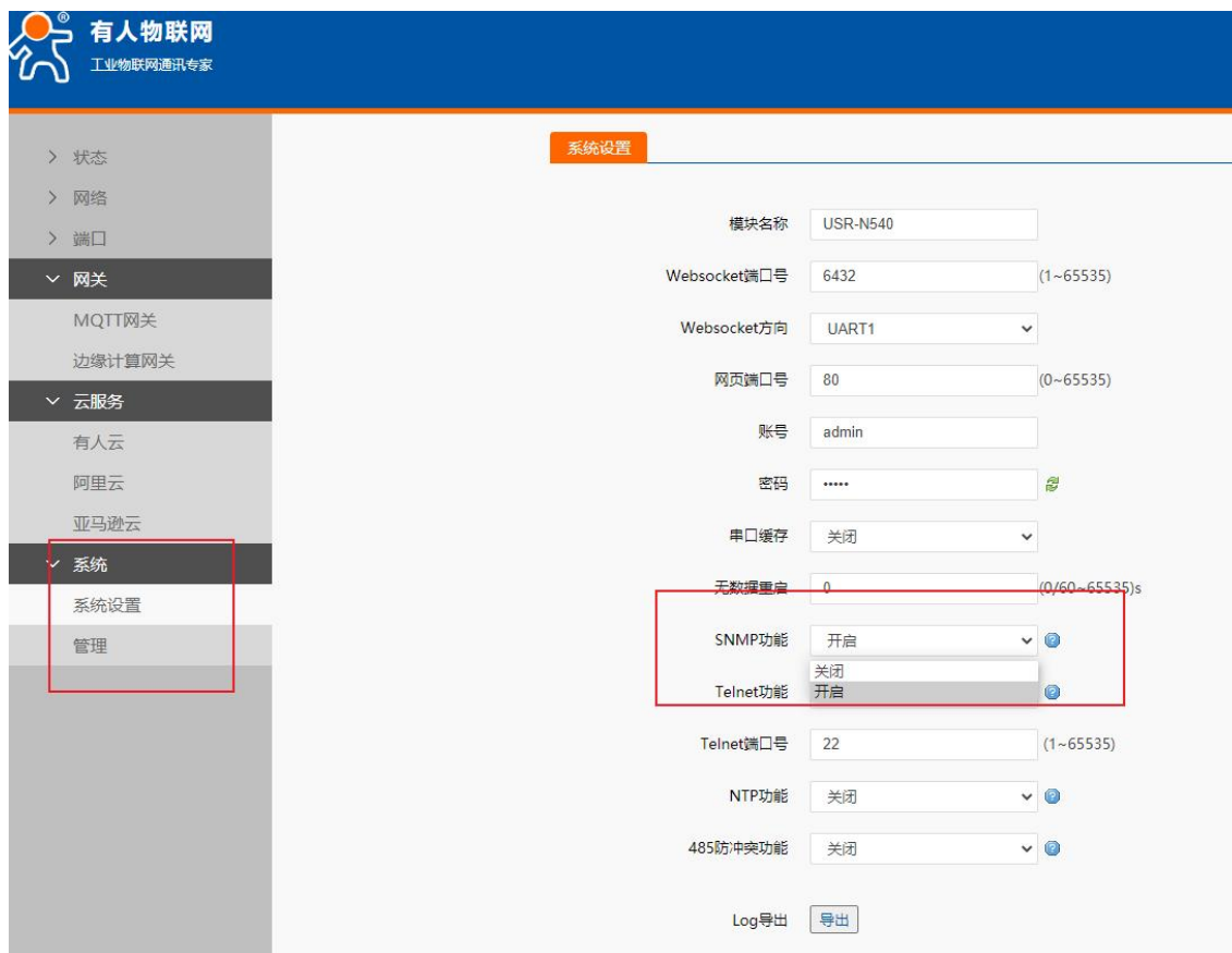
图 75 SNMP 状态网页开启
