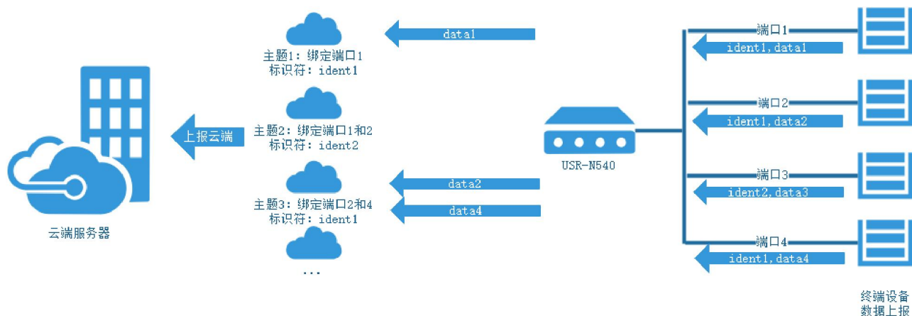
图 112 主题分发功能框图
