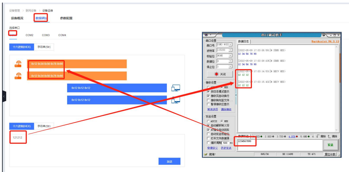
图 125 实现数据透传
