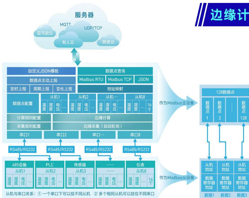
图 139 边缘计算功能框图
