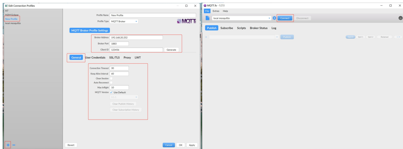
图 99 MQTT.fx 配置
