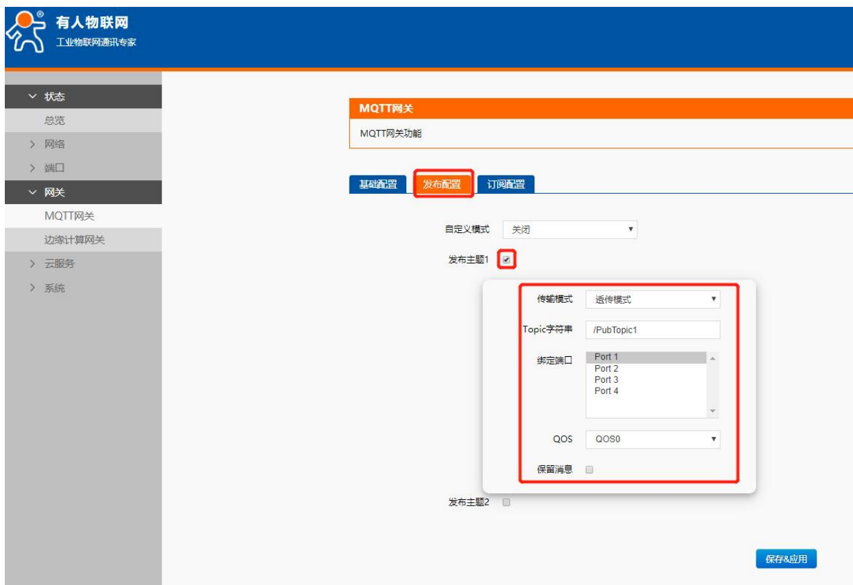
图 92 发布参数配置
