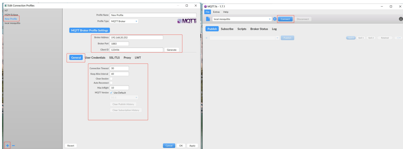
图 94 MQTT.fx 基础配置
