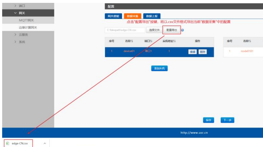
图 141 配置导出示意图
