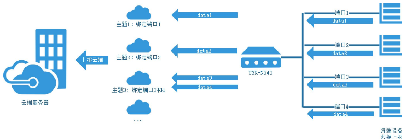
图 111 主题发布功能框图
