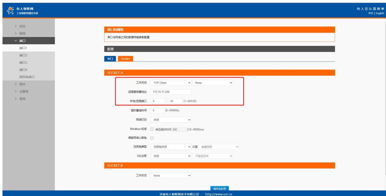
图 15 TCP Client 网页设置
