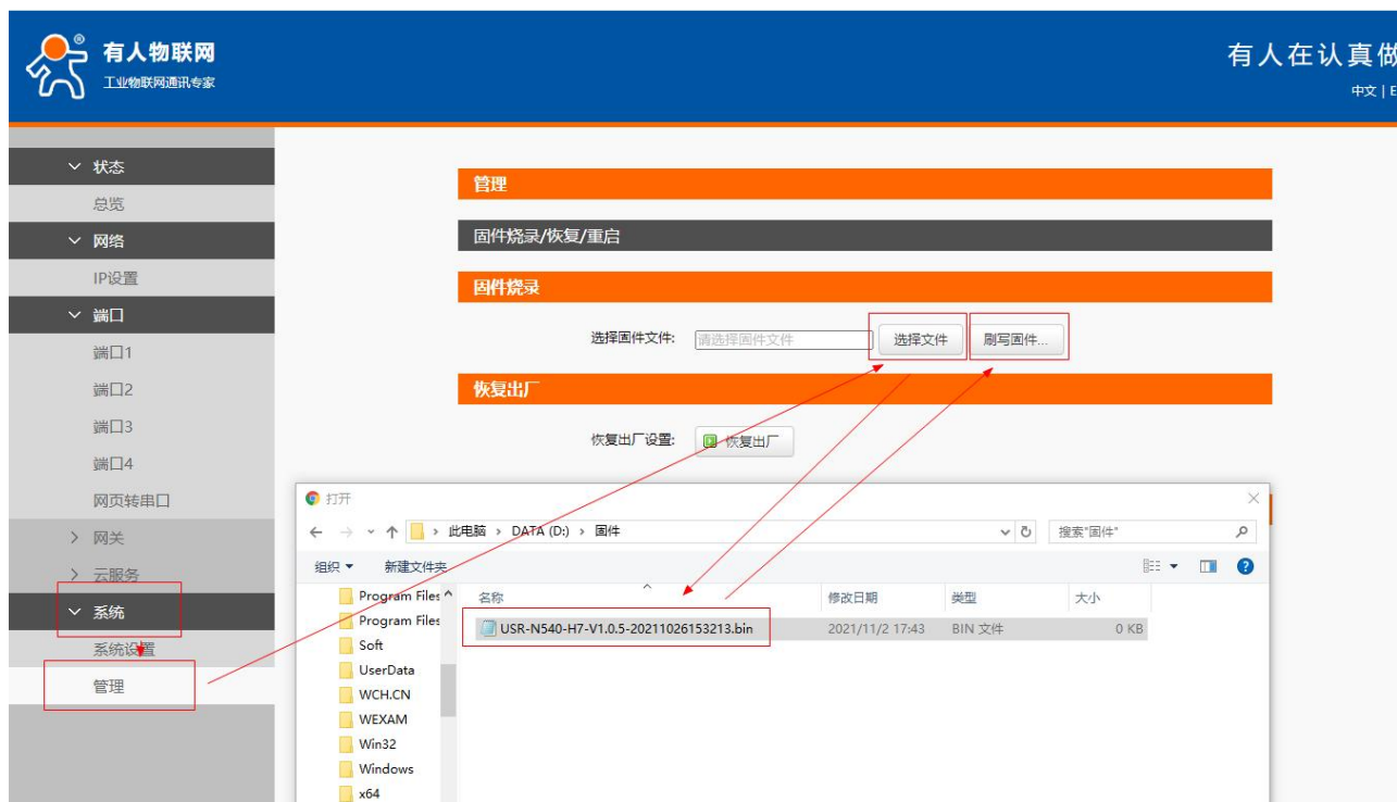
图 11 网页固件升级
