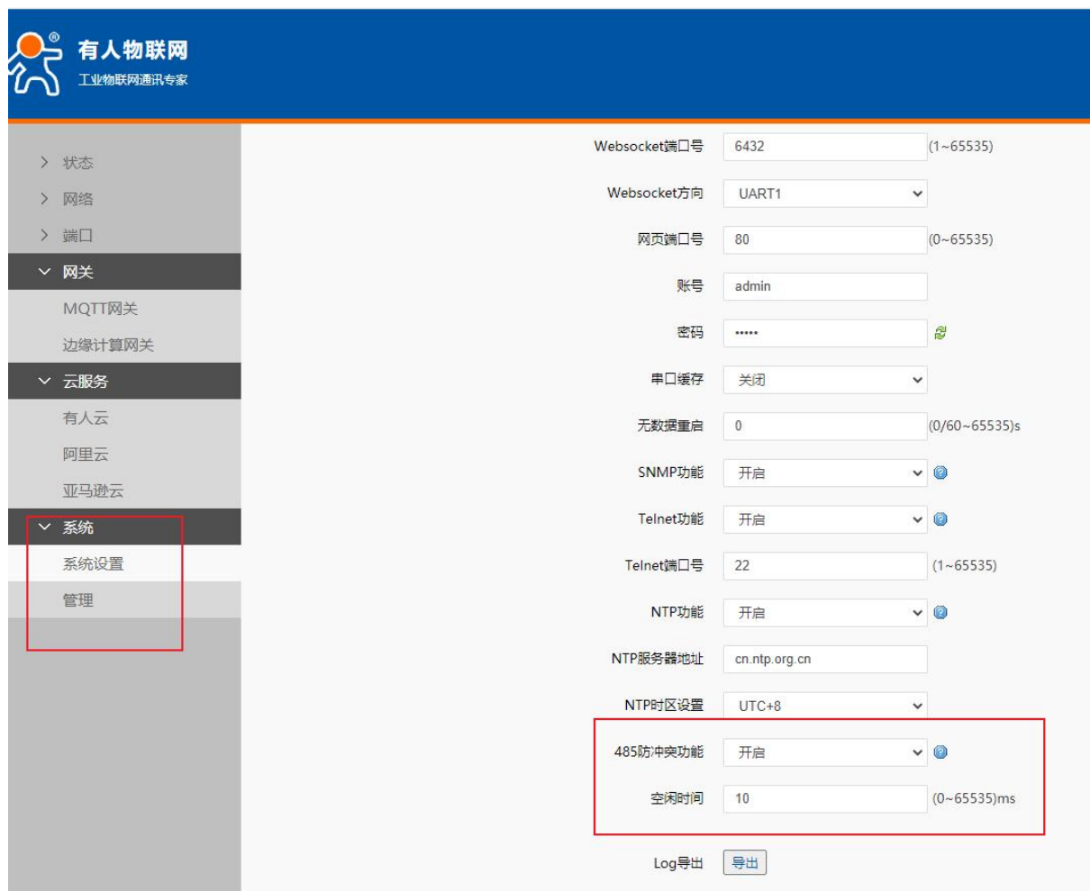
图 84 网页进行 485 防冲突配置
