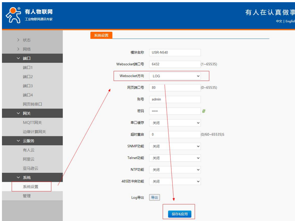
图 39 Websocket 方向设置 LOG
