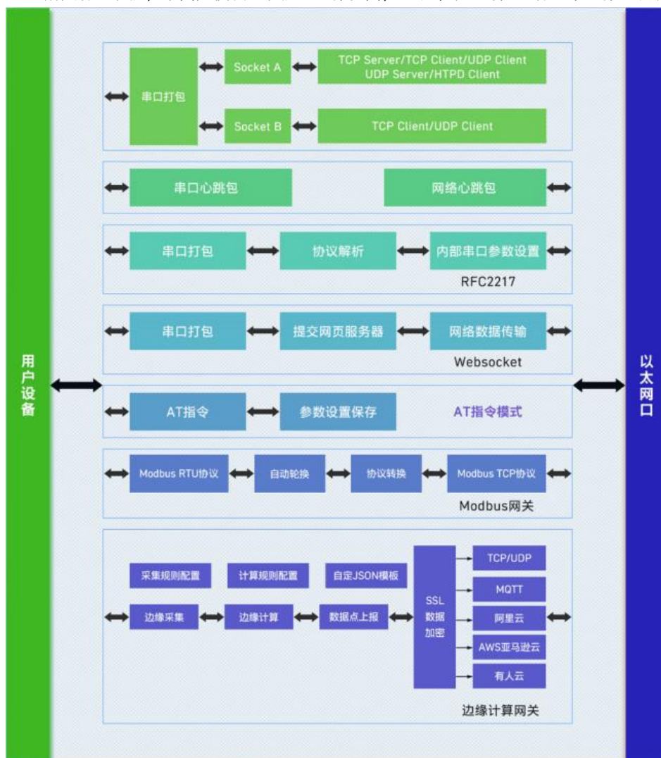
图 6 N5X0 功能框图
