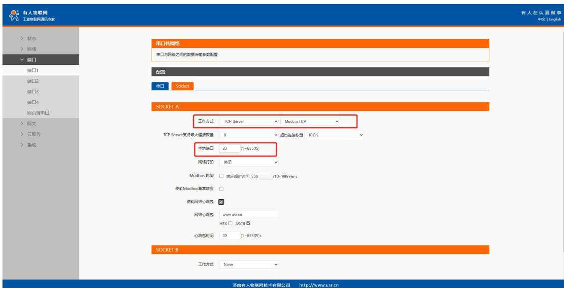
图 57 Modbus RTU 转 Modbus TCP
