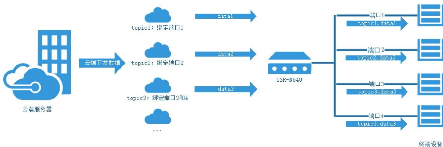
图 109 主题下发功能框图
