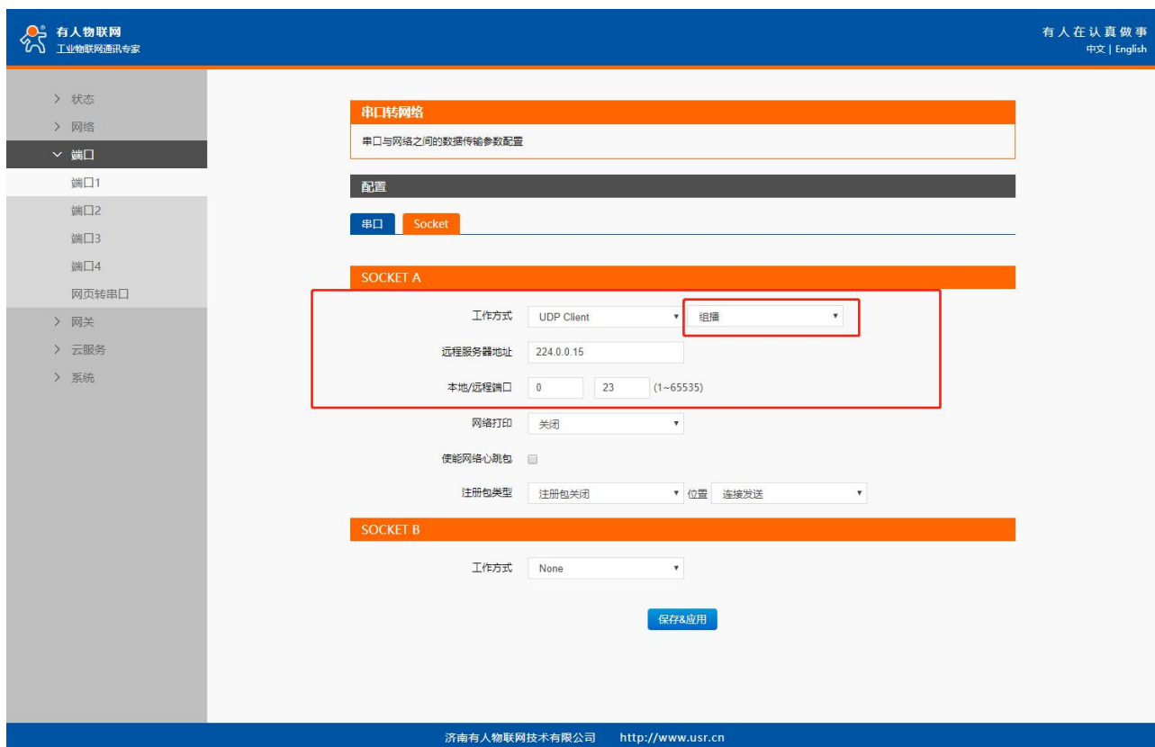
图 26 网页参数设置
