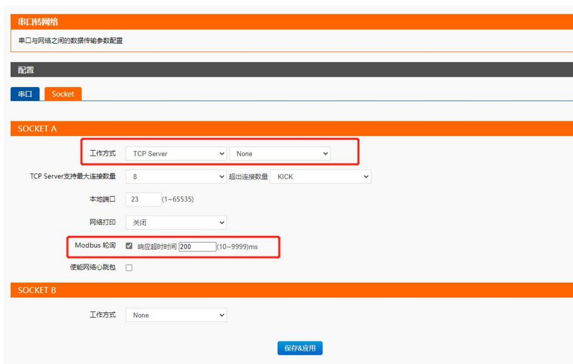
图 64 Modbus 轮询网页设置截图
