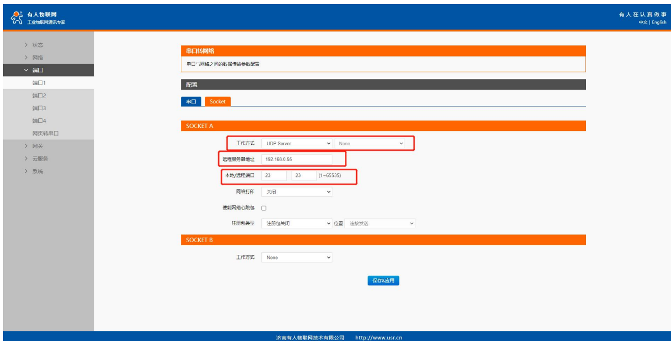
图 30 UDP Server 网页设置图
