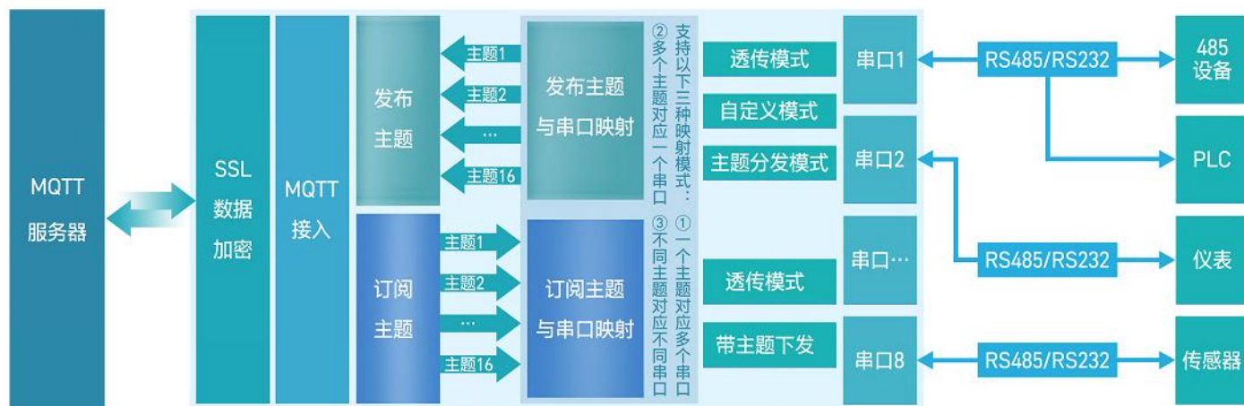
图 89 MQTT 功能框图
