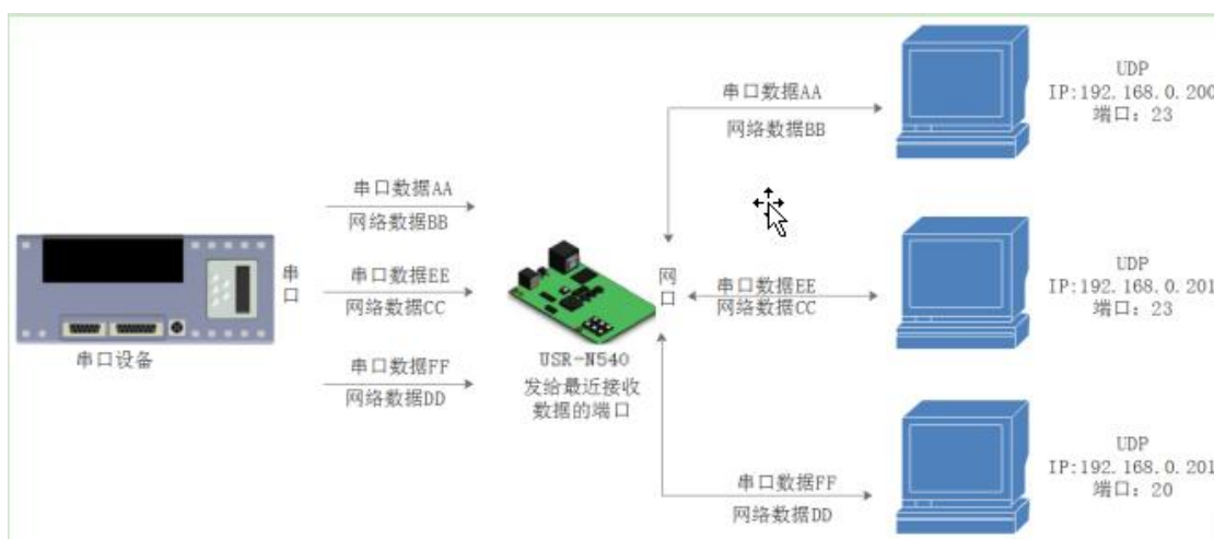
图 29 UDP Server 模式说明
