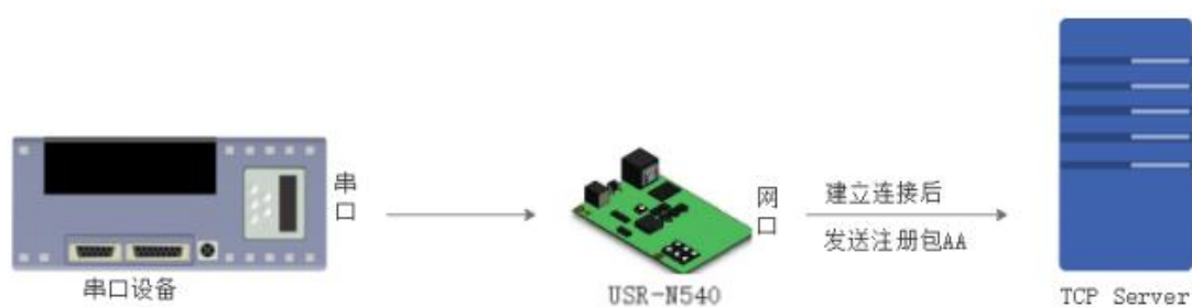
图 52 注册包建立连接发送注册包
