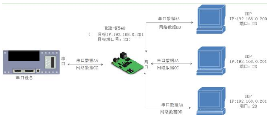
图 23 UDP Client 模式说明
