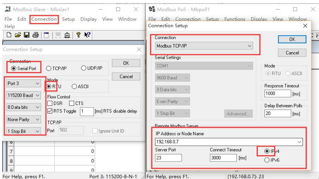
图 58 Modbus RTU 转 Modbus TCP 软件设置截图
