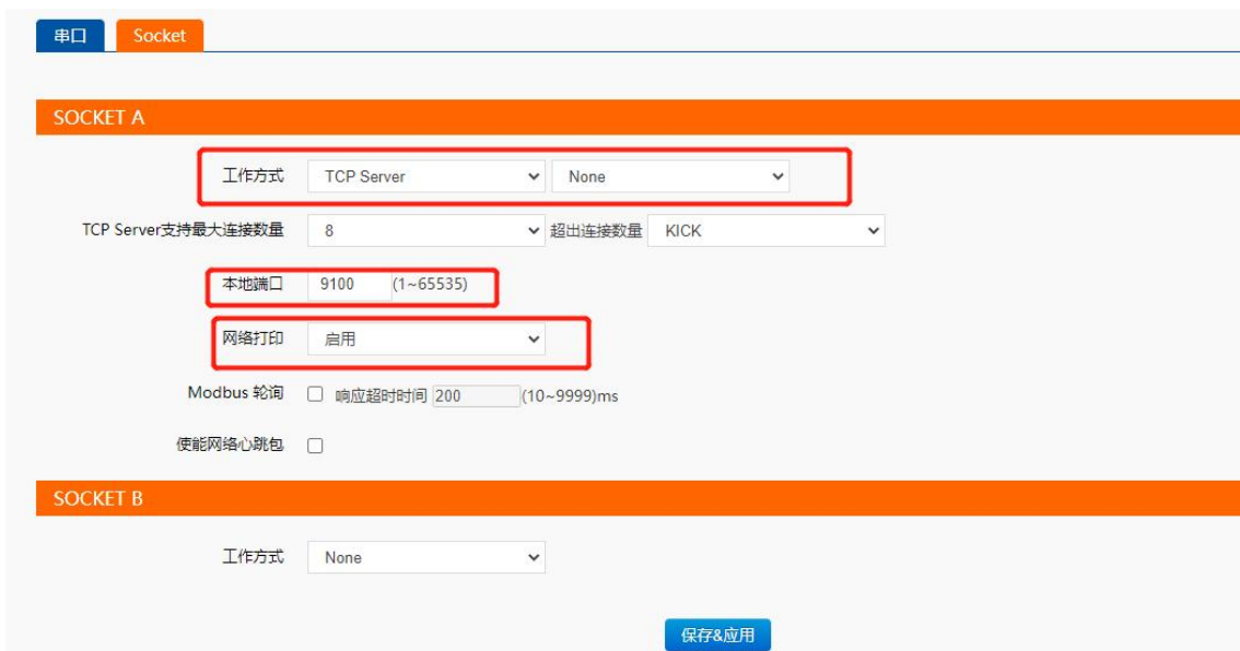
图 69 网络打印网页设置截图
