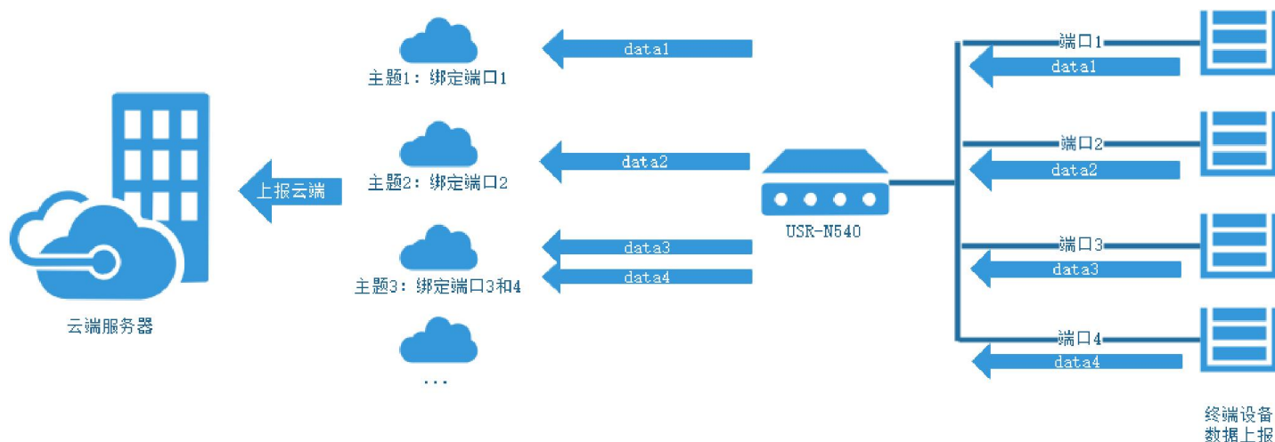
图 101 自定义数据发布模式功能框图
