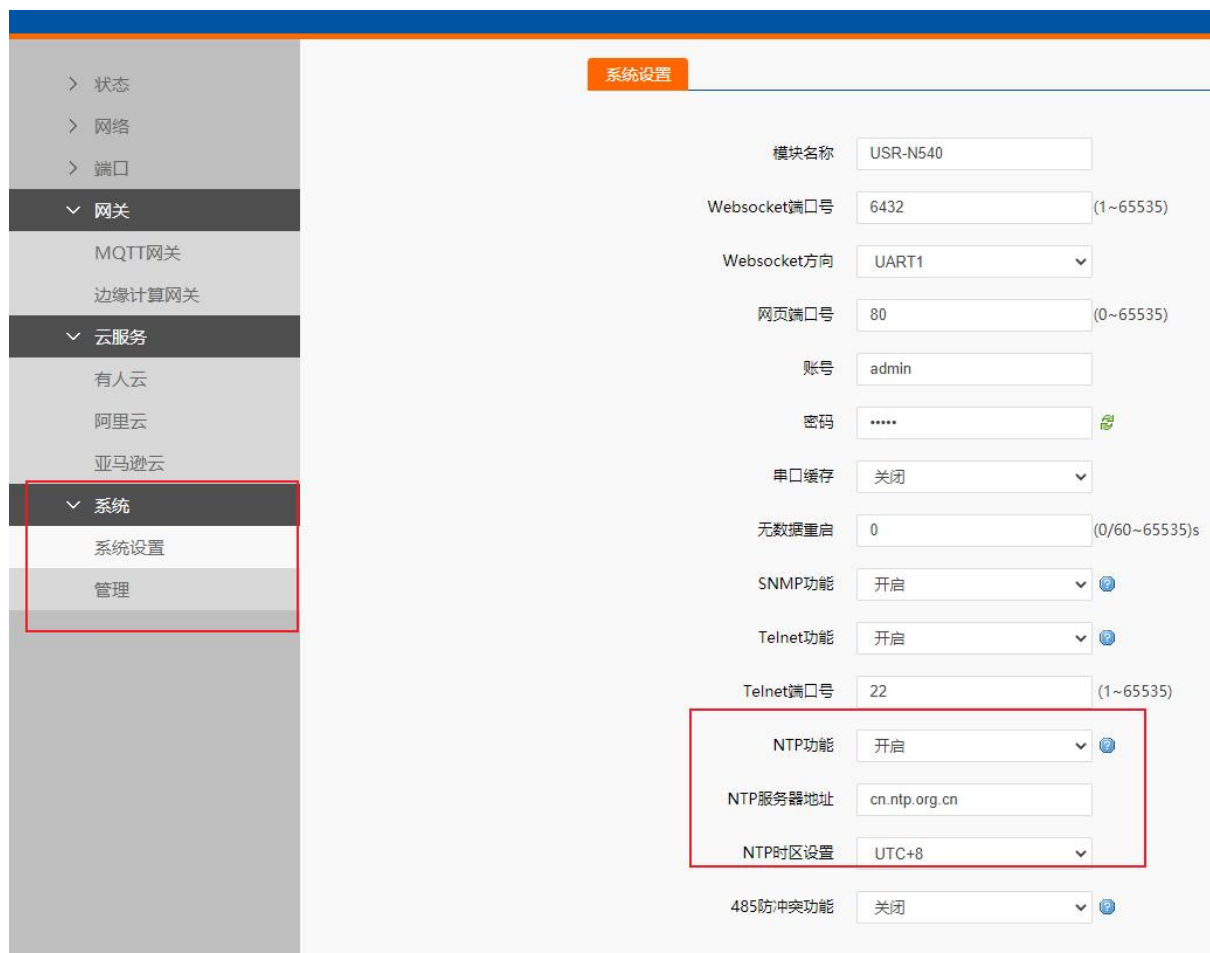
图 83 网页配置 NTP 功能开启
