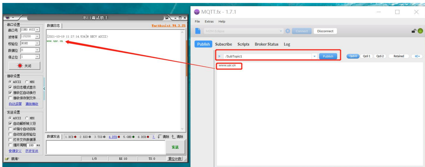
图 108 主题订阅数据透传测试
