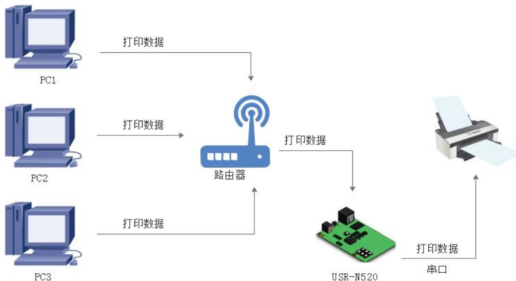
图 68 网络打印功能
