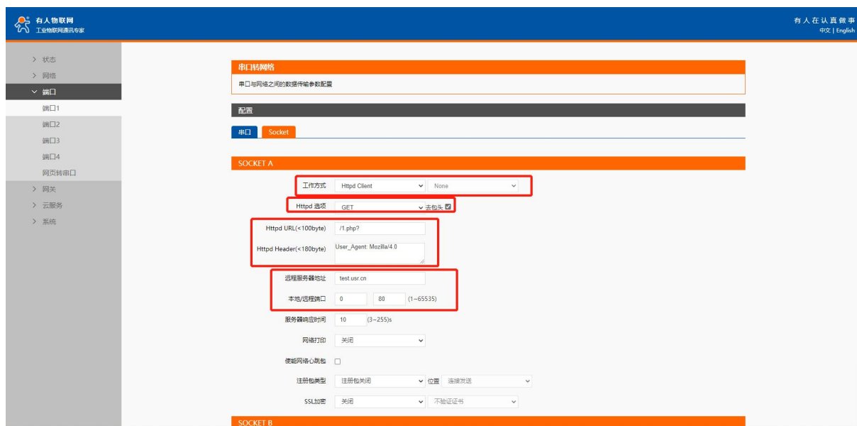
图 33 HTTPD Client 网页设置截图
