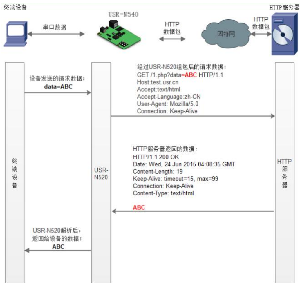
图 32 Httpd Client 模式说明
