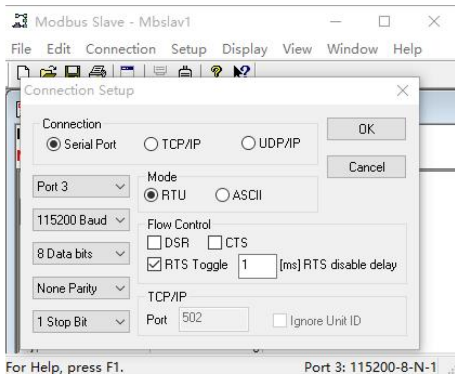
图 61 Modbus RTU 主动查询设置截图
