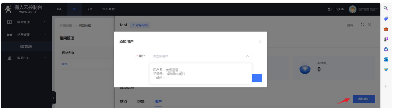
图 11 添加用户
