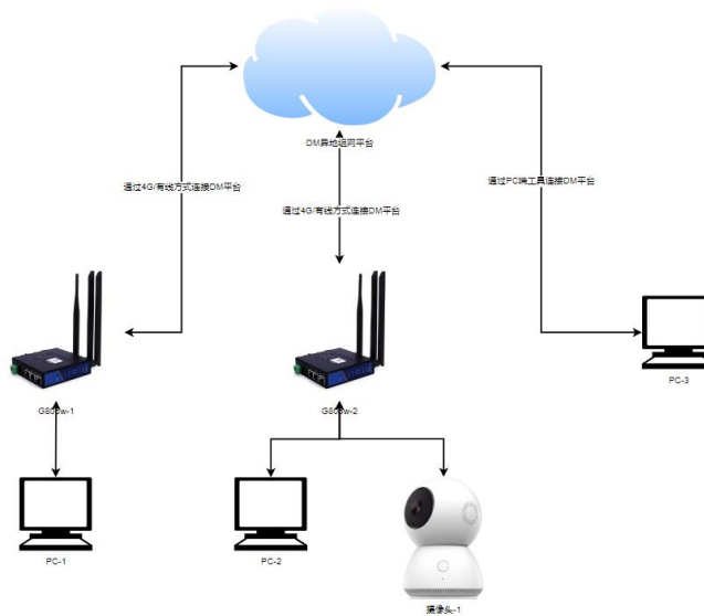
图 5 组网拓扑
